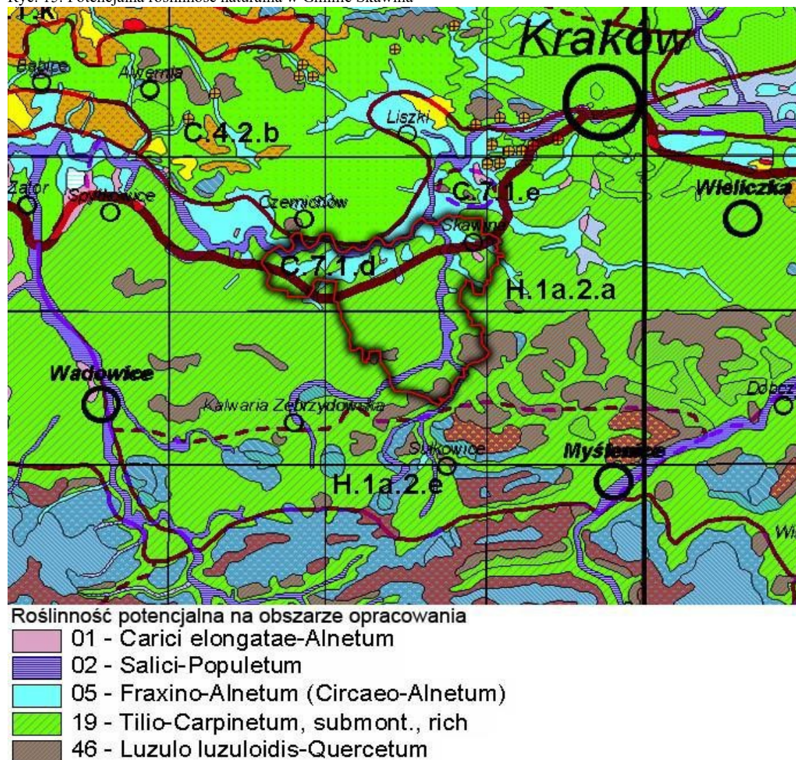
Ryc. 15. Potencjalna roślinność naturalna w Gminie Skawina
