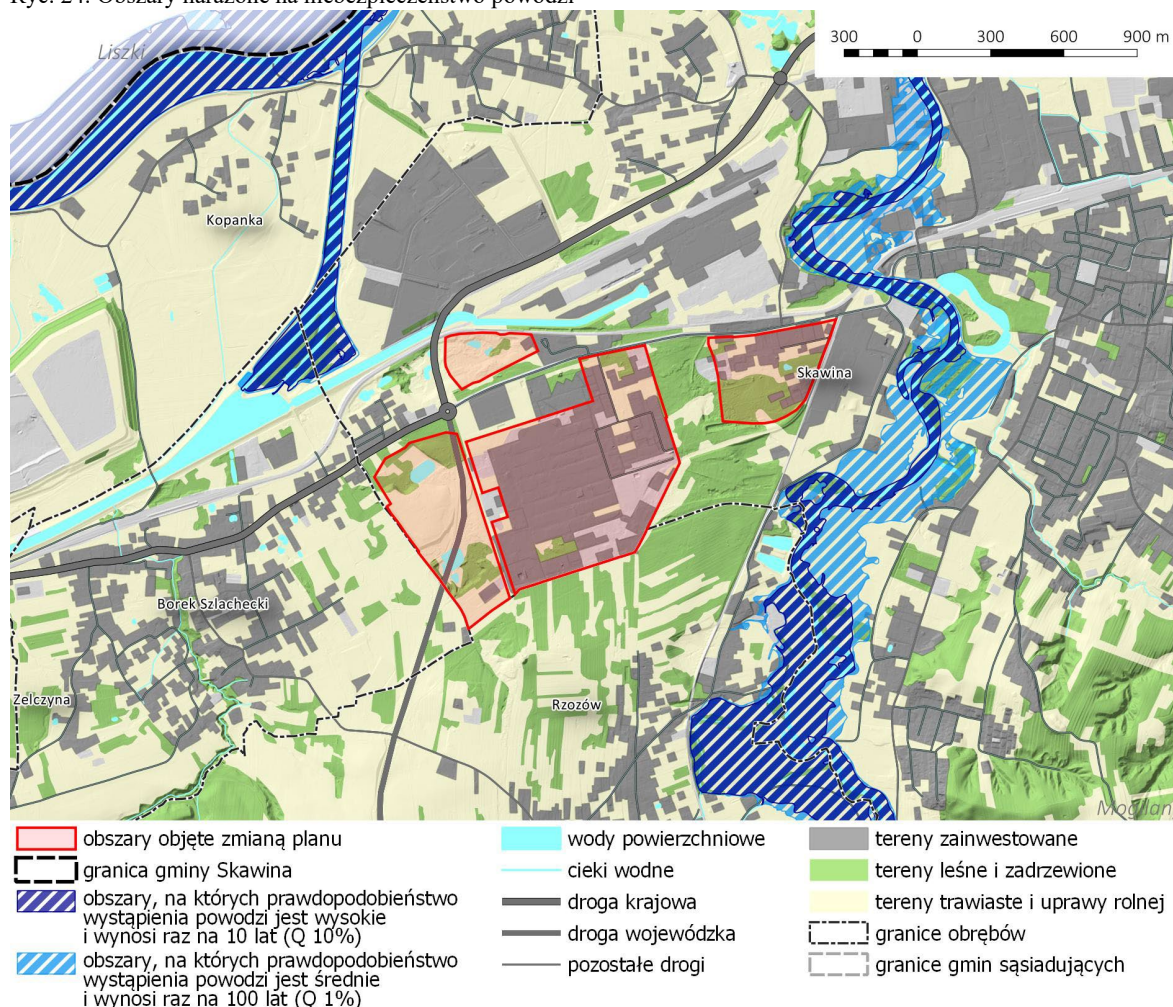
Ryc. 24. Obszary narażone na niebezpieczeństwo powodzi
