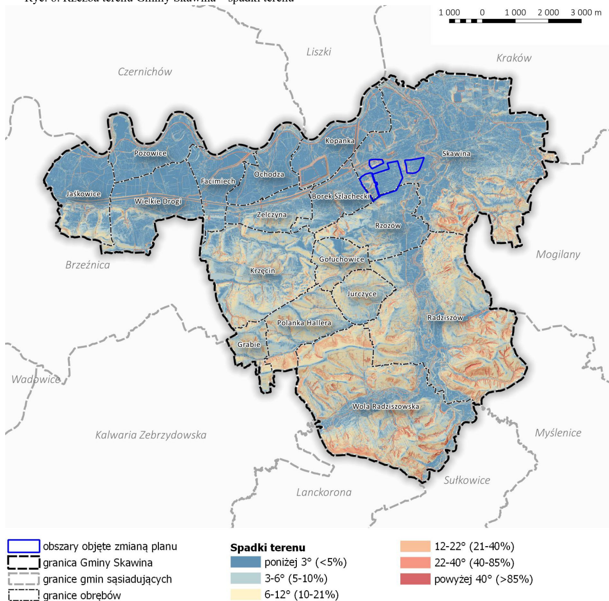
Ryc. 6. Rzeźba terenu Gminy Skawina – spadki terenu
