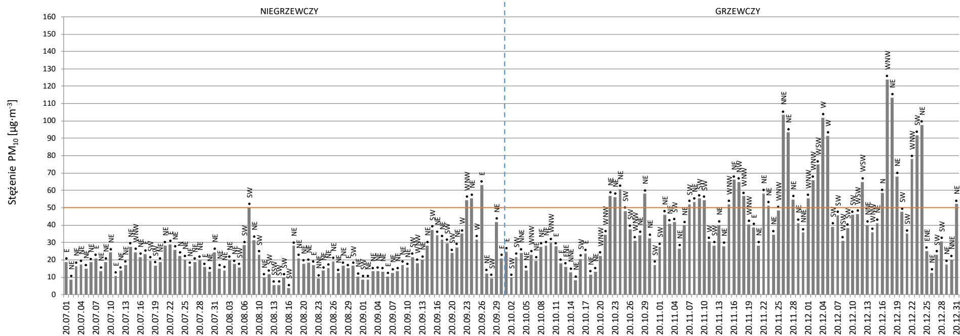
Rysunek 6. Przebieg serii stężeń dobowych pyłu PM 10 z zaznaczonymi kierunkami wiatru – punkt pomiarowy w Skawinie, okres: 1.07–31.12.2020 r.
