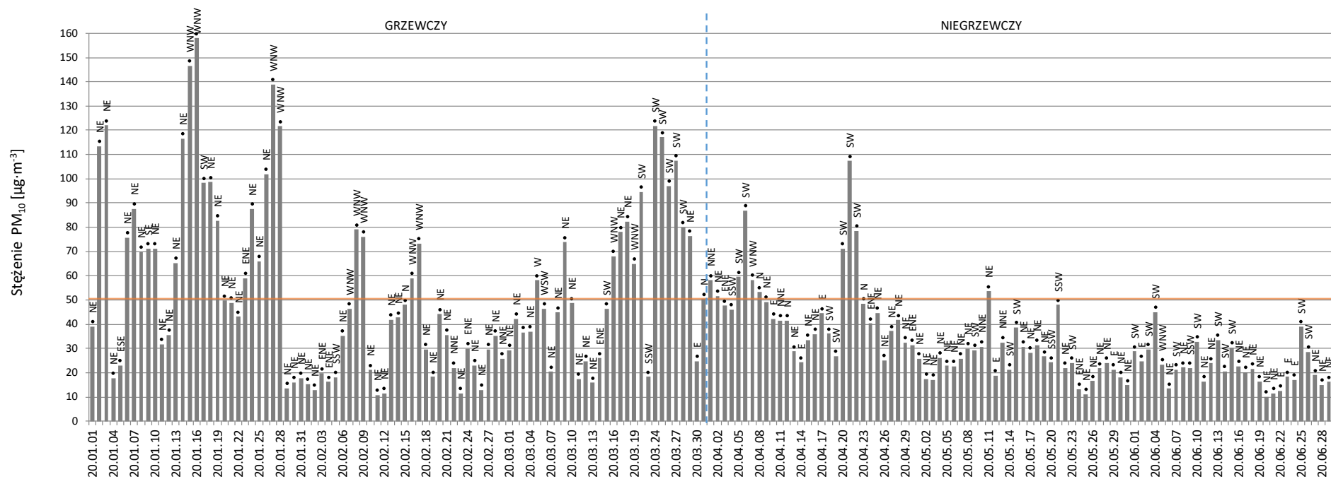
Rysunek 5. Przebieg serii stężeń dobowych pyłu PM 10 z zaznaczonymi kierunkami wiatru – punkt pomiarowy w Skawinie, okres: 1.01-30.06.2020 r.
