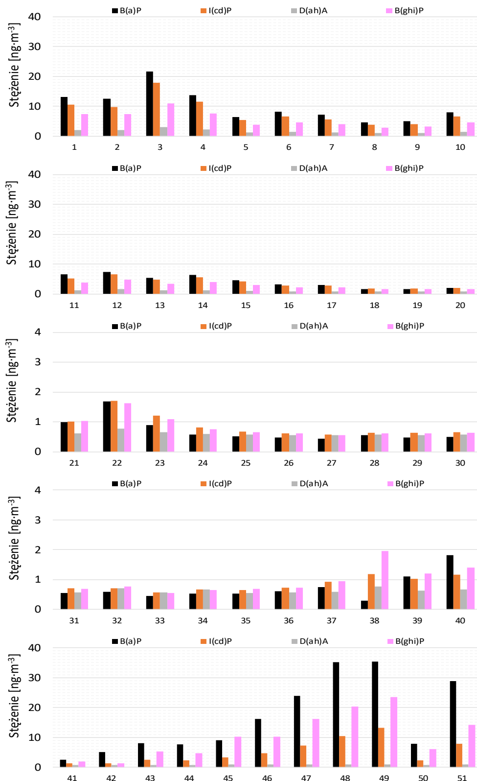
Rysunek 13. Stężenie wybranych WWA [ng·m -3 ] (benzo(a)piren, indeno(123-cd)piren, dibenzo(ah)antracen, benzo(ghi)perylen) w próbkach tygodniowych pyłu PM 10 ze Skawiny (okres: 01.01–21.12.2020 r.)
